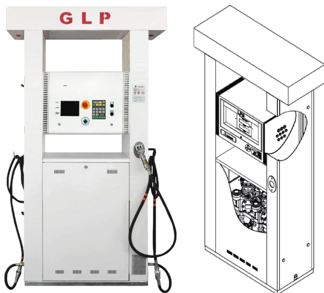
Dispensador de GLP 1 producto 2 mangueras con 1 y 2 CPU's marca Yenen
