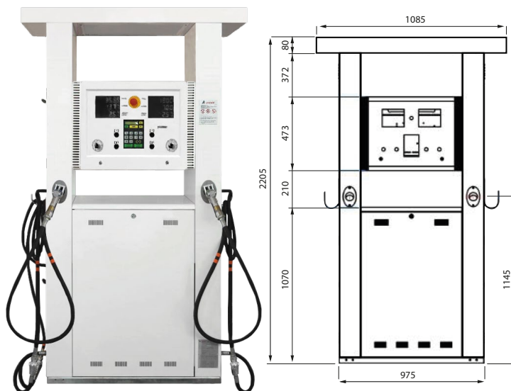
Dispensador de GLP 1 producto 4 mangueras con 2 CPU's marca Yenen
